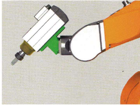
傾斜法蘭45°
