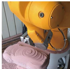
雕刻
